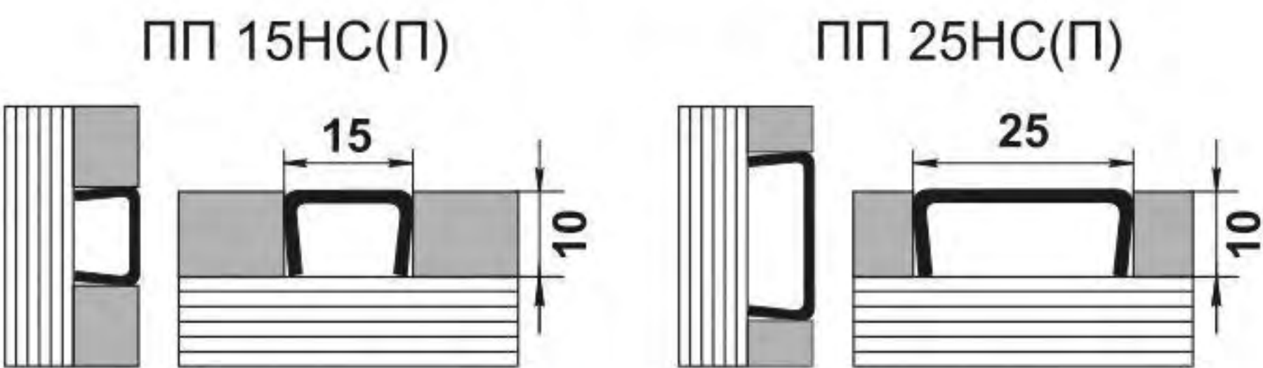
Бордюр-вставка
